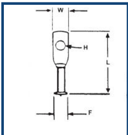
Acoustical Hanger (Lagging Stud)
